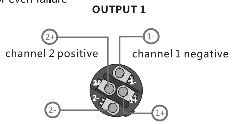
OUTPUT 1
