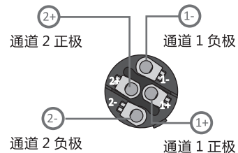
功率输出 1
