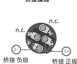
功率输出 1 桥接模式
