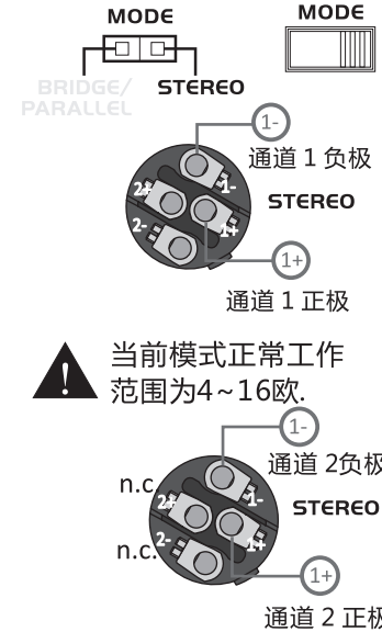
SPEAKON 功率输出 - 扬声器输出 NL4 Speakon 接线方式
