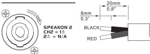
SPEAKON 功率输出 - 扬声器输出 NL4 Speakon 接线方式
